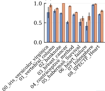
(e) AUC
