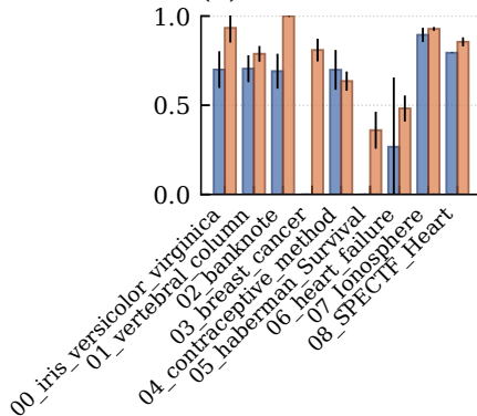
(b) Precision
