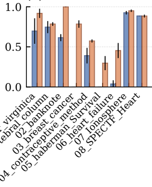
(d) F1
