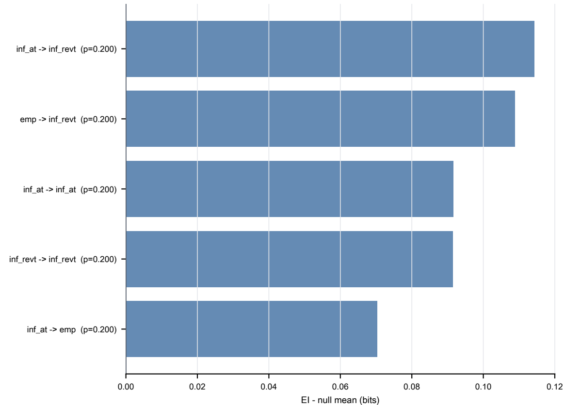
成对跨期边
