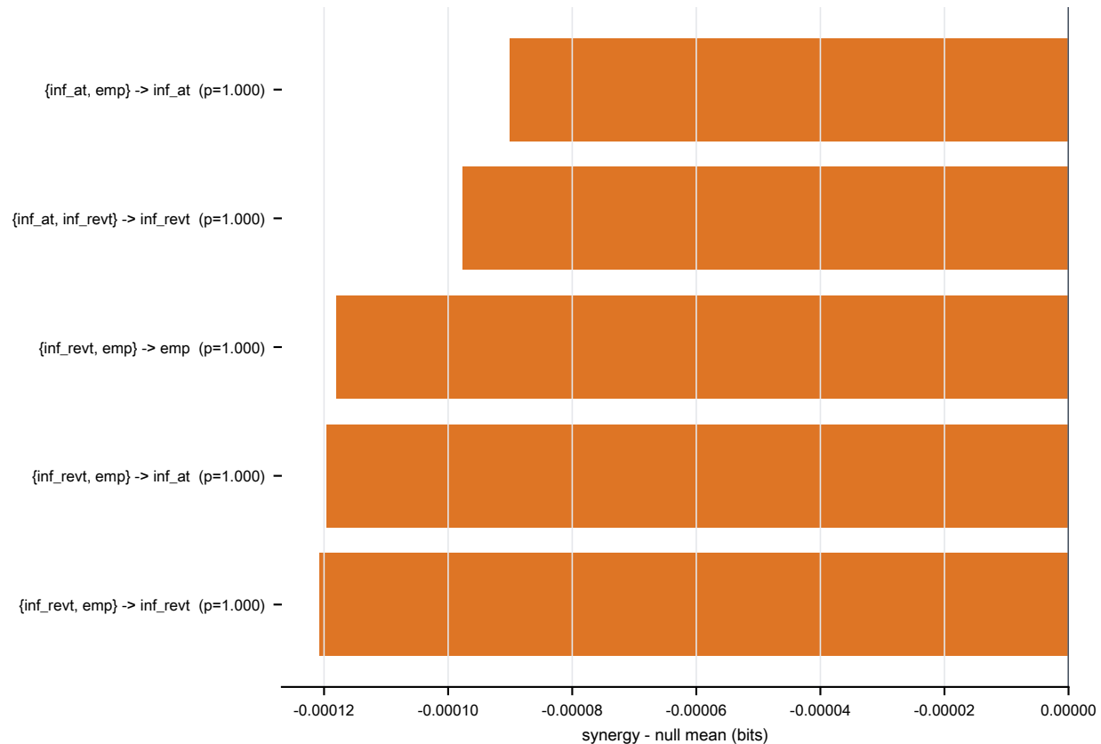
协同超边
