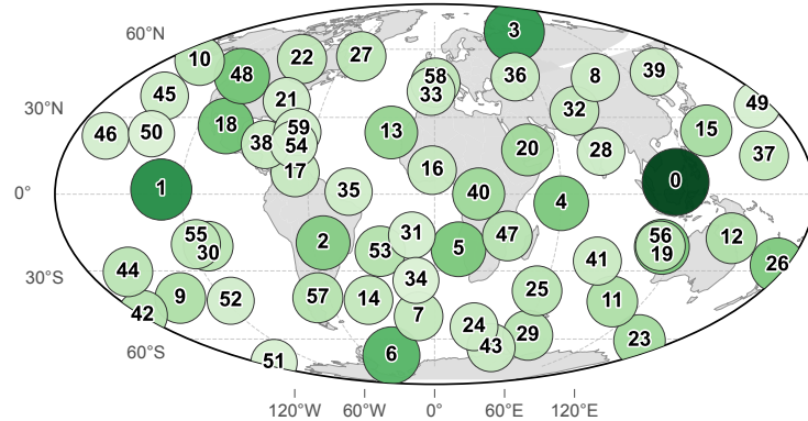
Multistep conditioned EI AMCE
