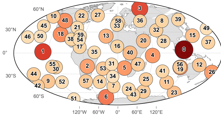
Multistep conditioned EI ACE
