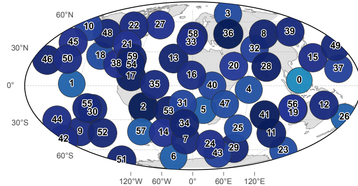
Multistep conditioned EI ACS
