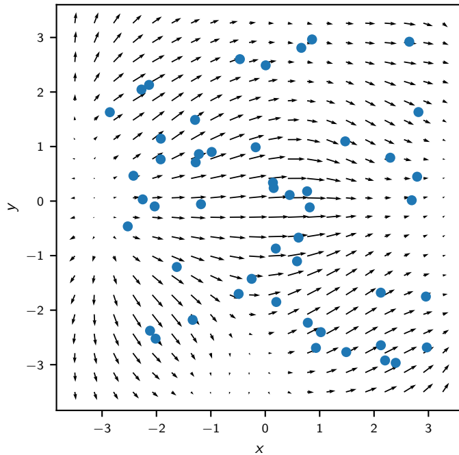
Posterior Mean Gradient (conditioned on \nabla f )
