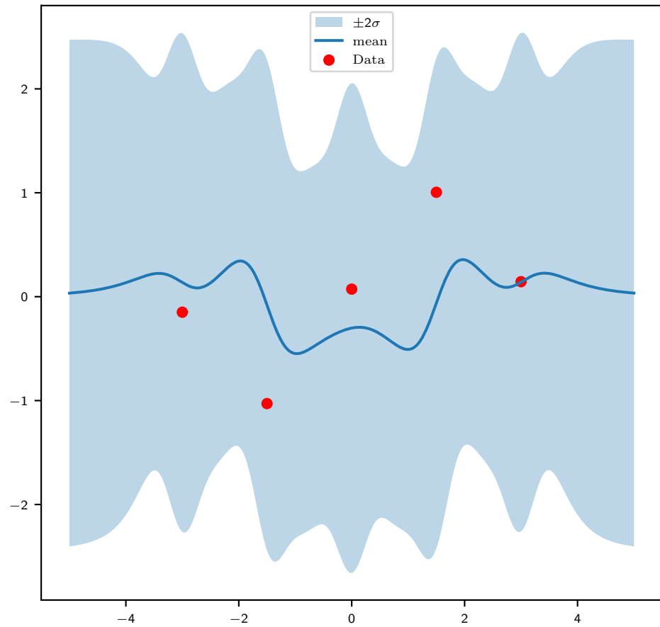
Posterior GP
