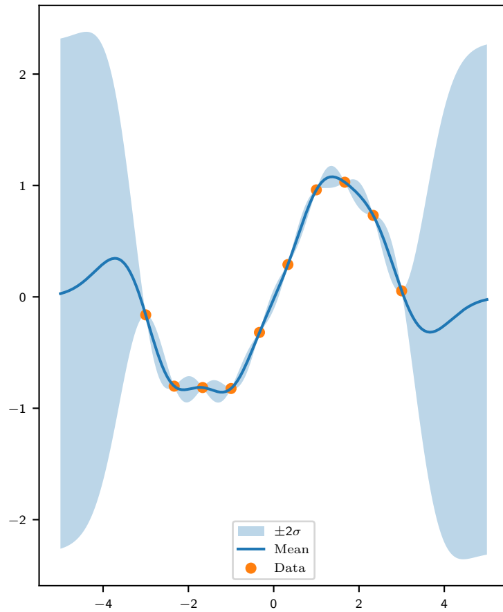
Posterior GP (latent f)
