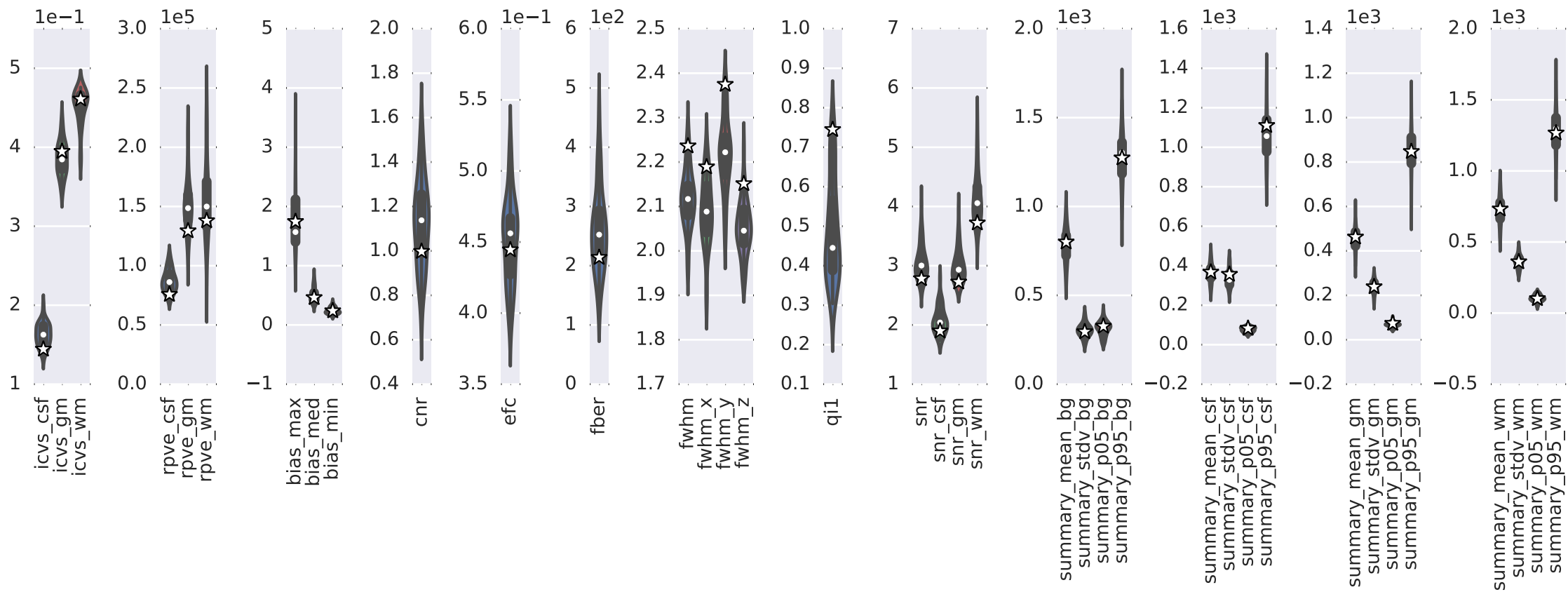
QC measures (subject sub-126_ses-FU)
