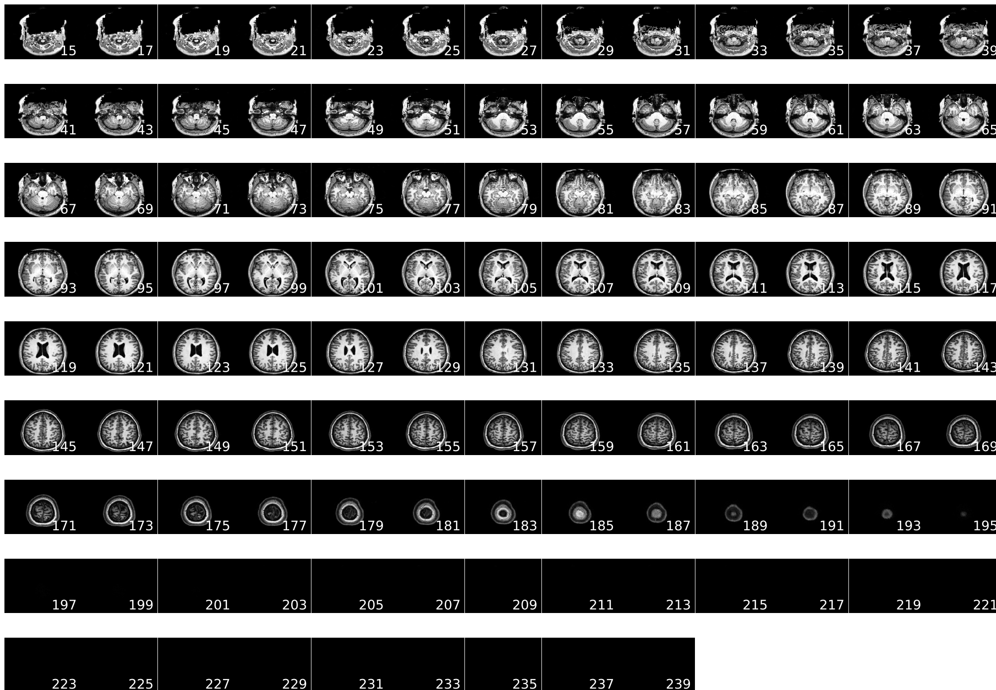
Volume, subject sub-126 (ses-BL_T1w)
