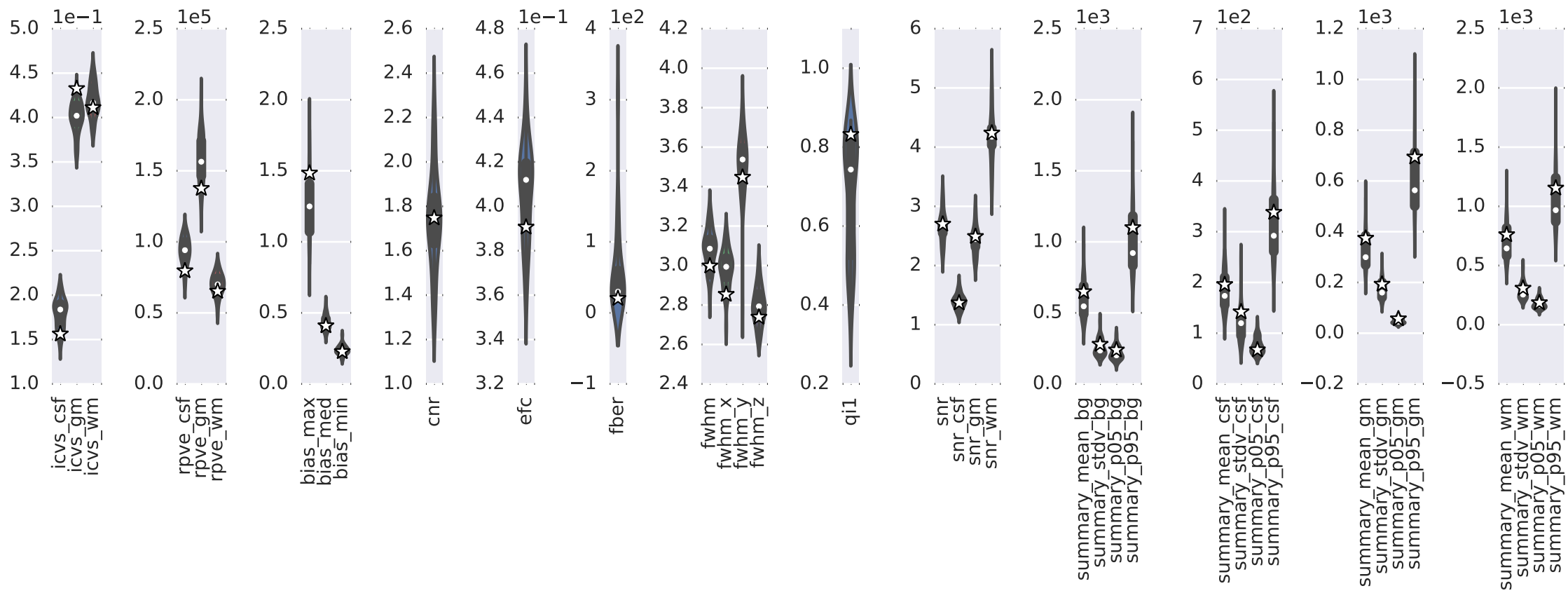
QC measures (subject sub-126_ses-BL)
