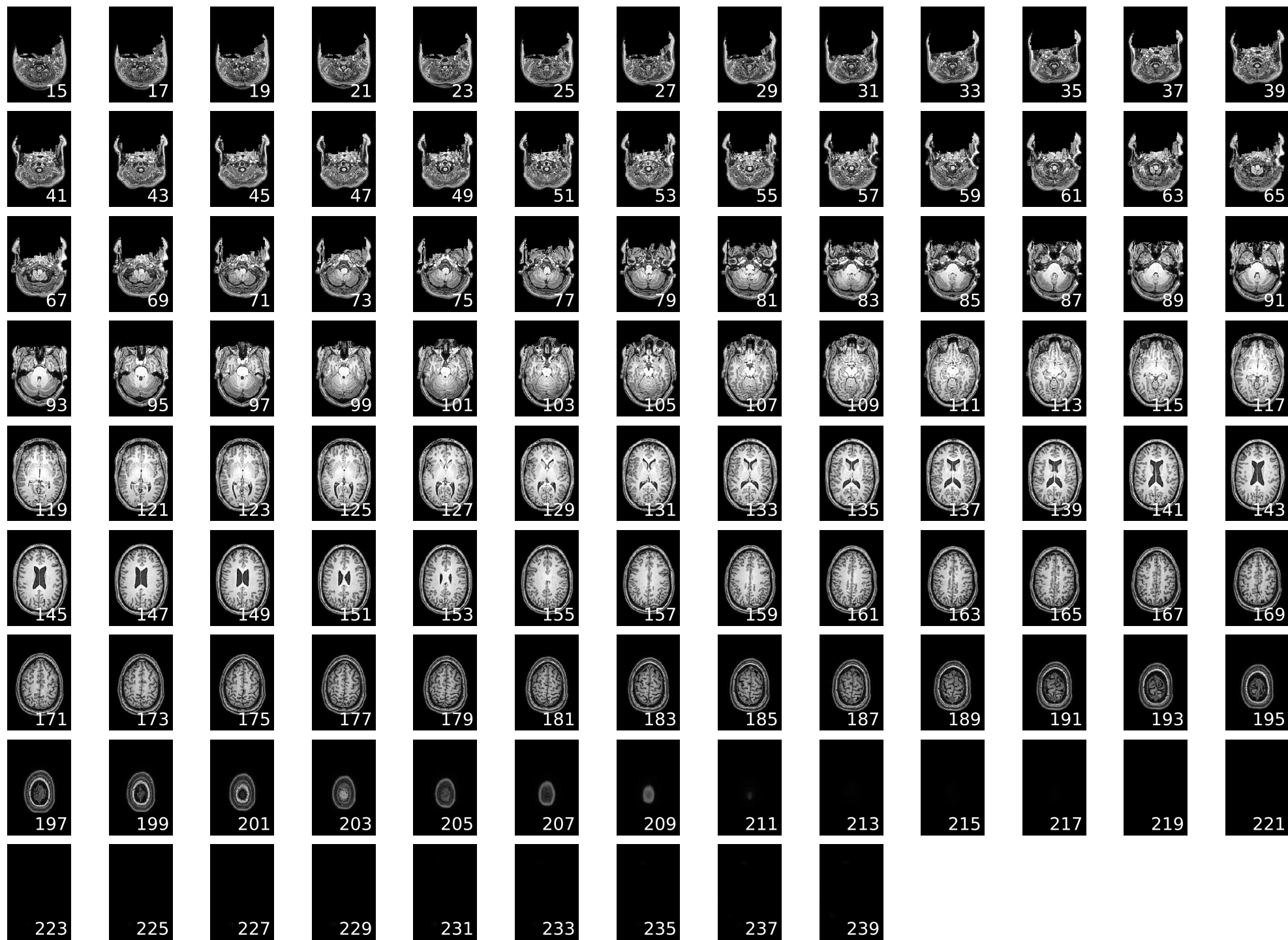
Volume, subject sub-126 (ses-FU_T1w)
