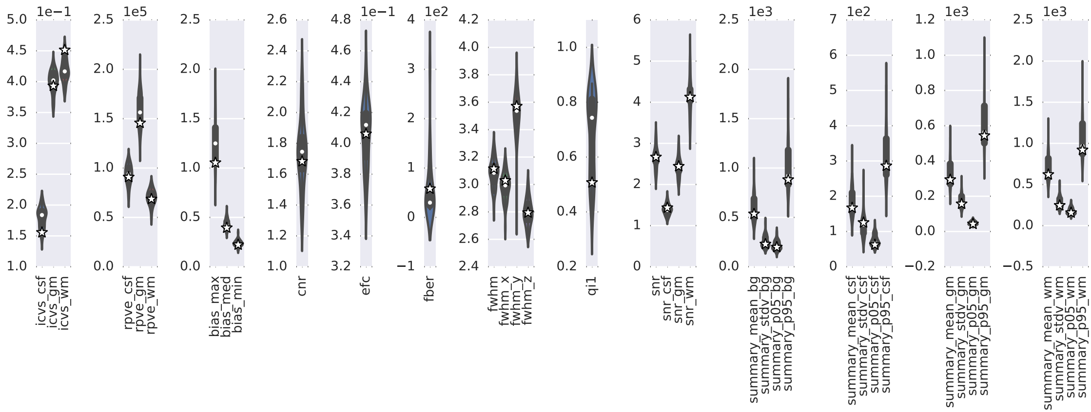
QC measures (subject sub-306_ses-BL)
