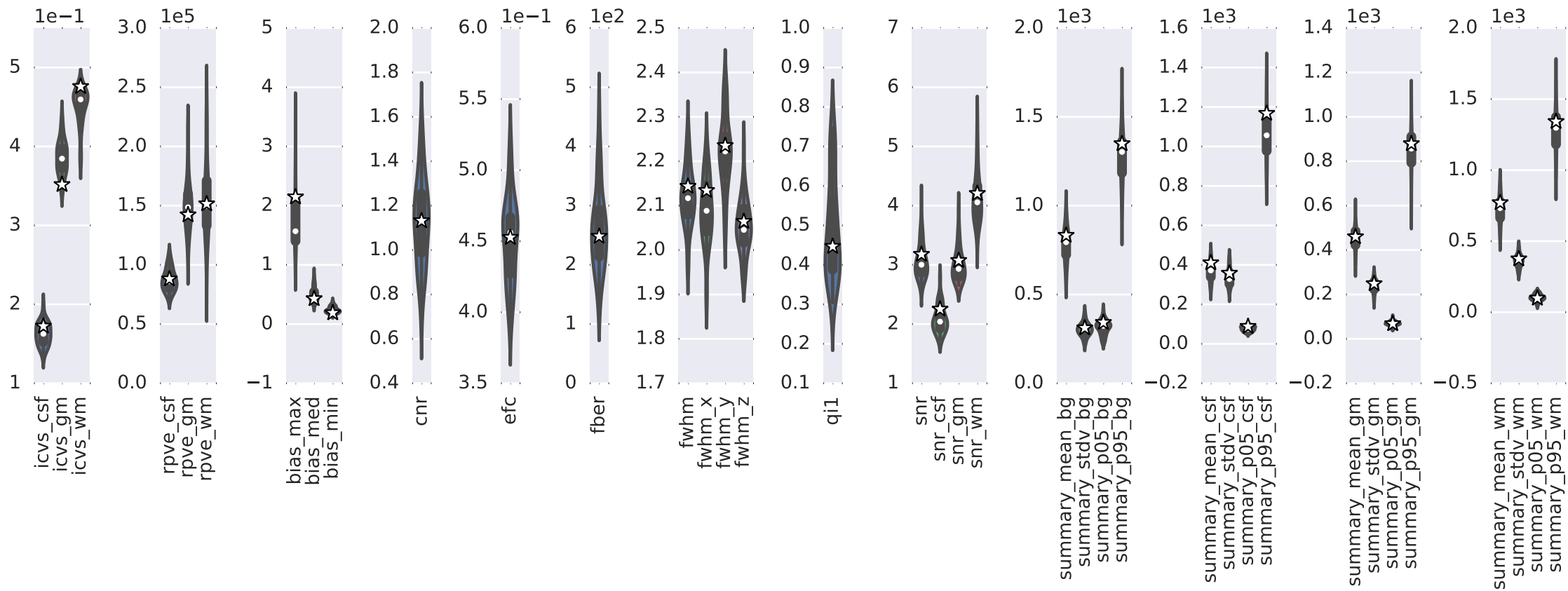
QC measures (subject sub-306_ses-FU)
