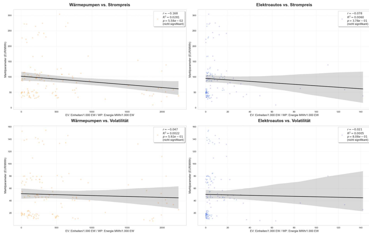
Korrelation: Wärmepumpen/Elektroautos vs. Strompreis/Volatilität (Jahresbasis, 2018-2024)
