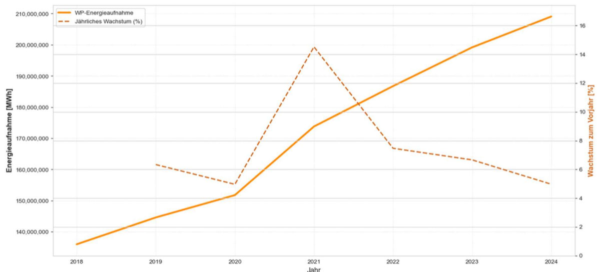
Wärmepumpen: Jährliche Energieaufnahme & Wachstumsrate
