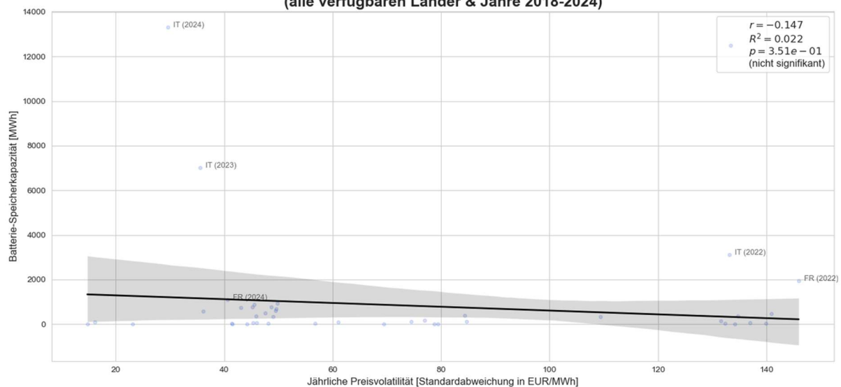
Korrelation: Preisvolatilität vs. Batterie-Speicherkapazität (alle verfügbaren Länder & Jahre 2018-2024)
