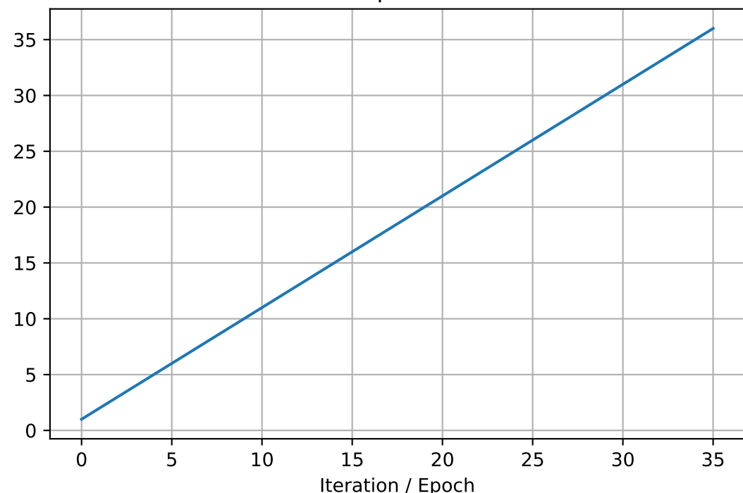
tau2
