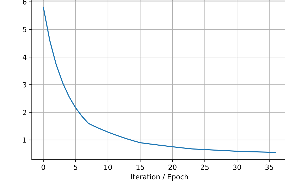
+1.9996e1 tau4_target_Eqf
