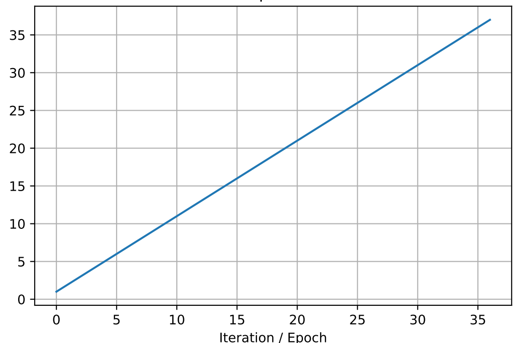
tau2
