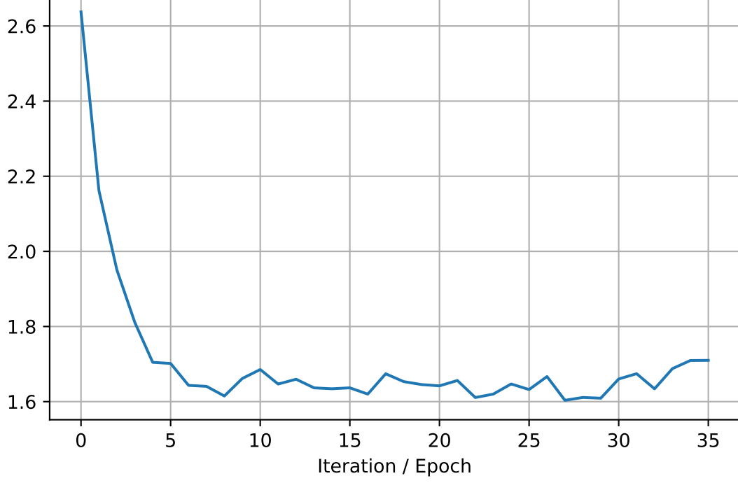
tau2_target_Eqf2
