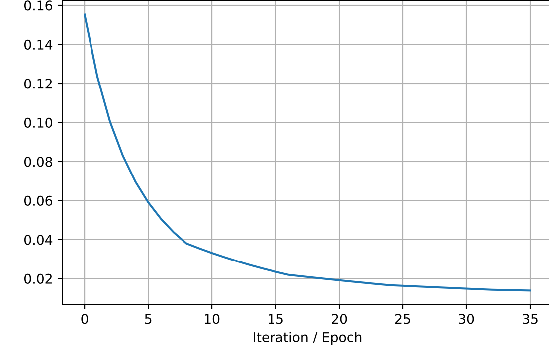
tau4_var
