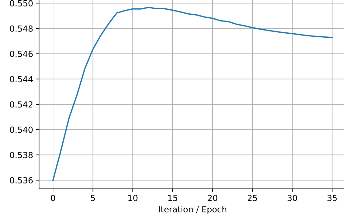
tau4_Eqf
