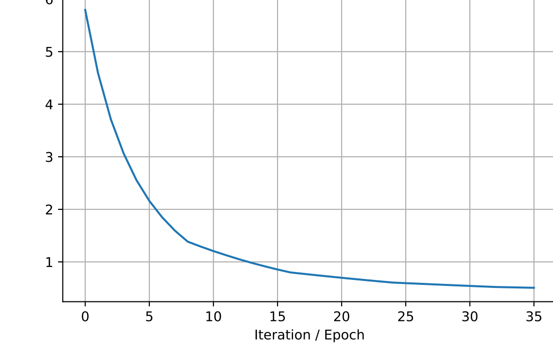
+1.9996e1 tau4_target_Eqf
