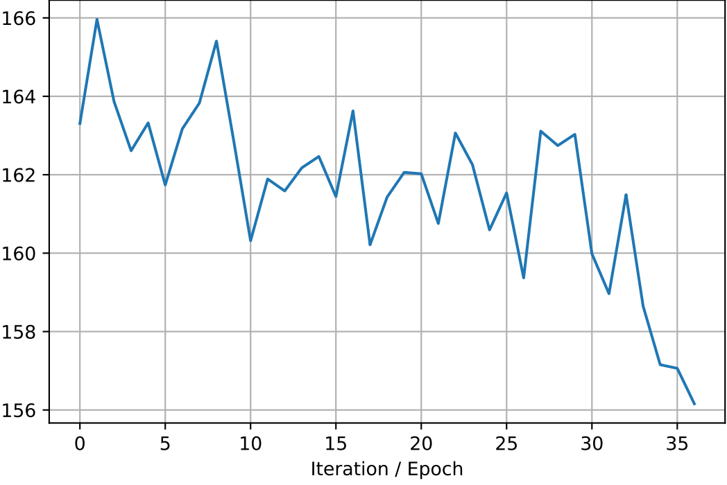
tau2_Eqf2
