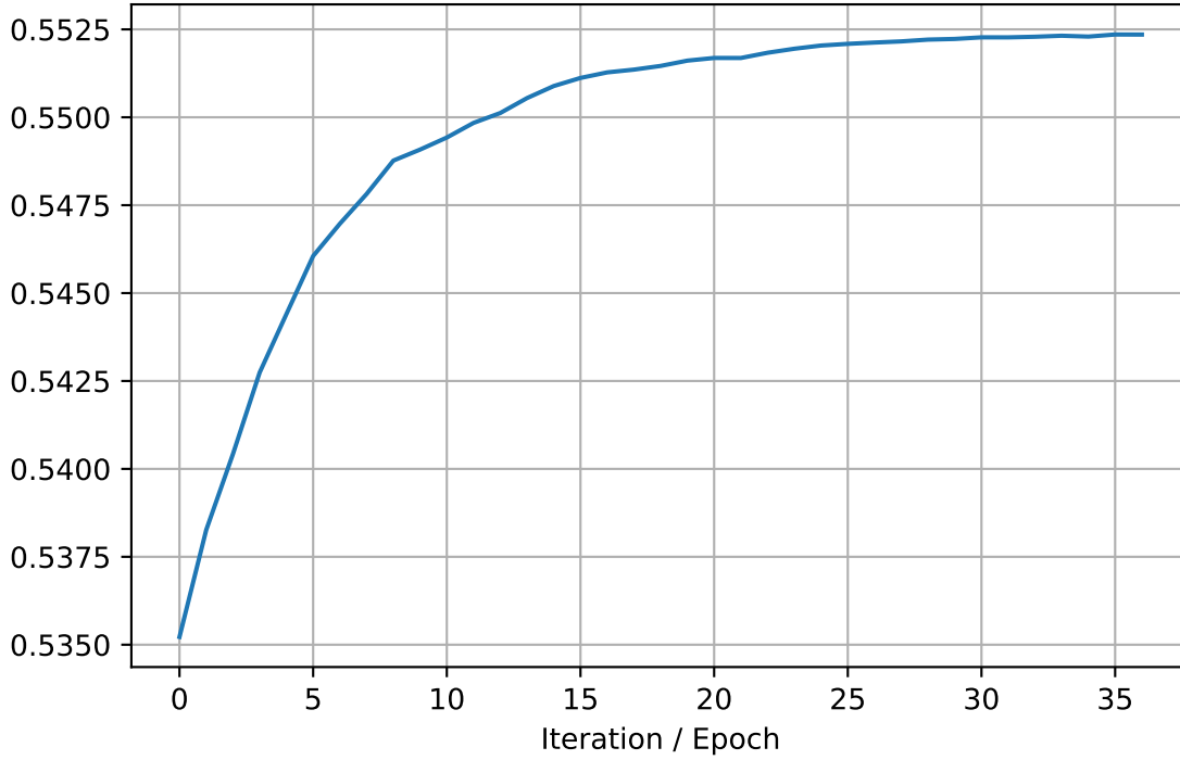
tau4_Eqf
