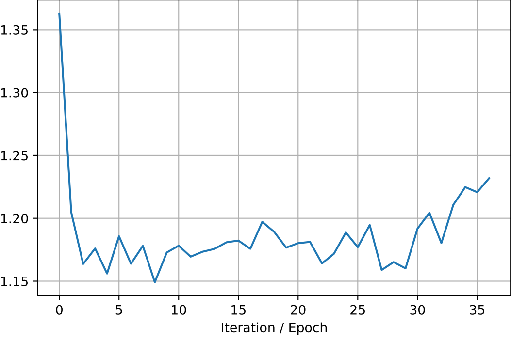
tau1_target_Eqf1
