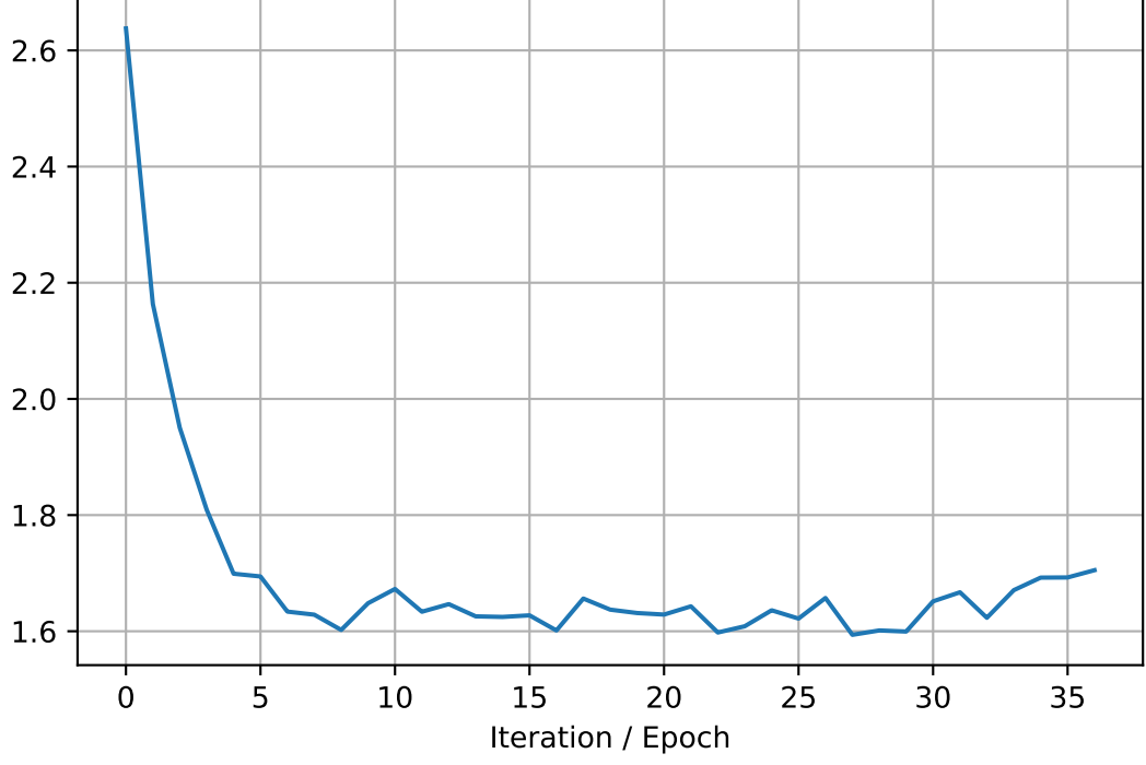
tau2_target_Eqf2
