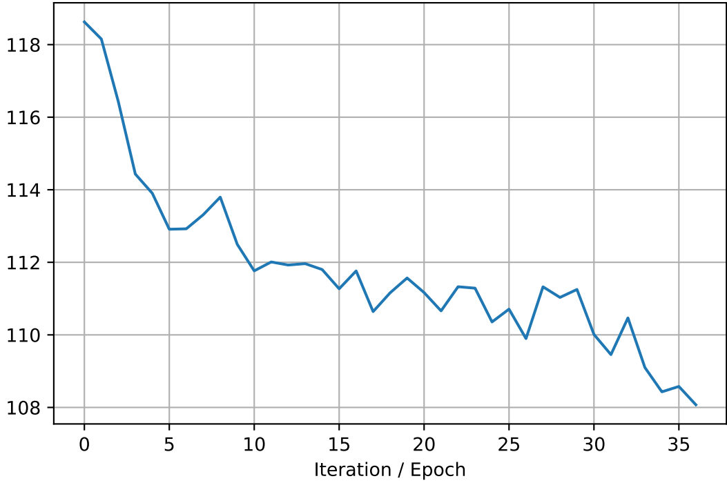
tau1_Eqf1
