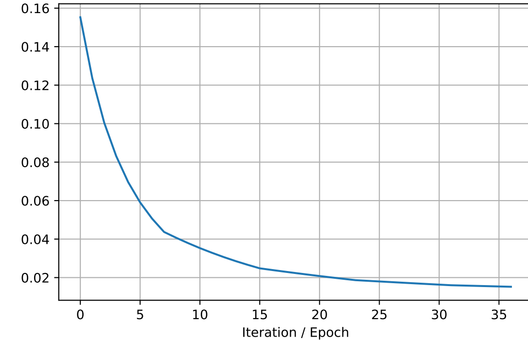
tau4_var
