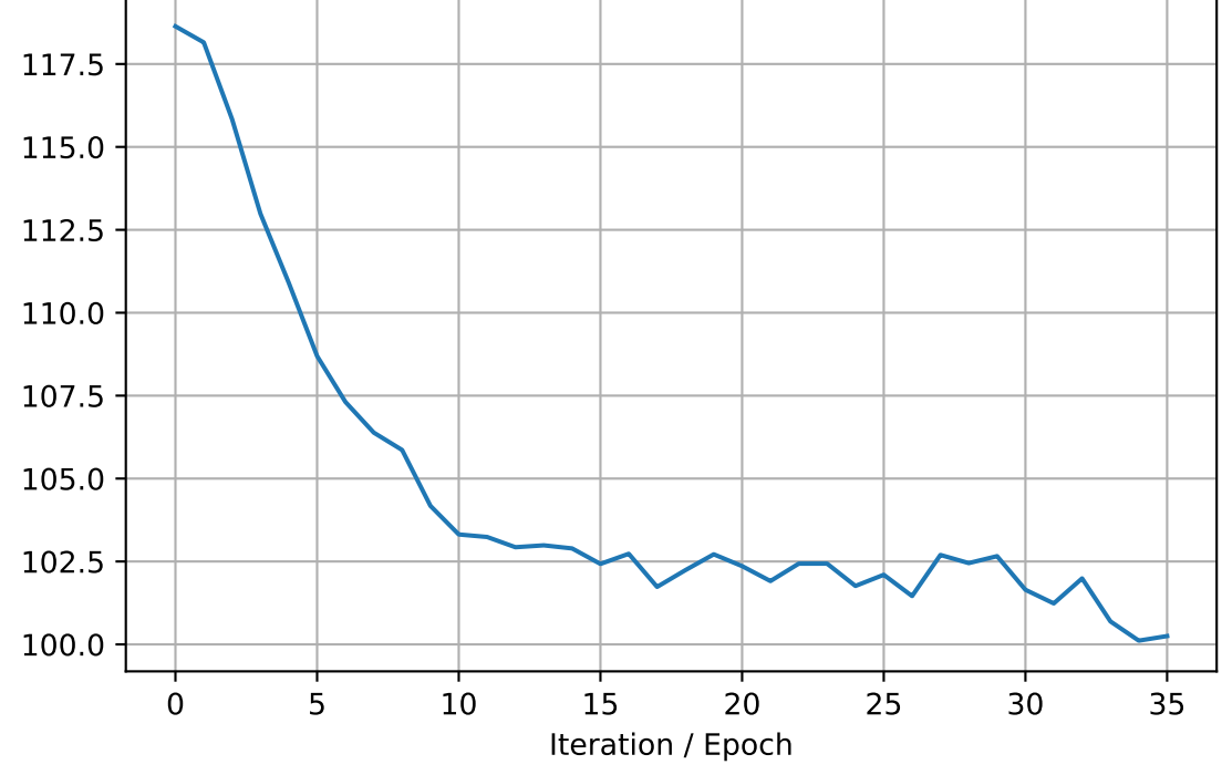
tau1_Eqf1
