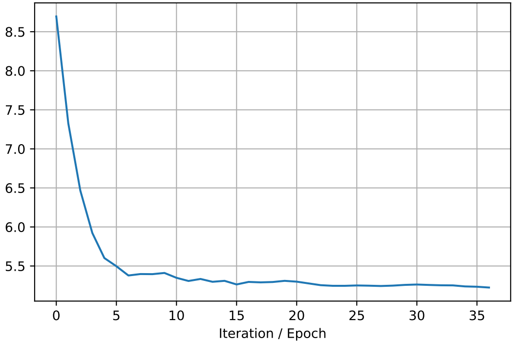
tau2_var
