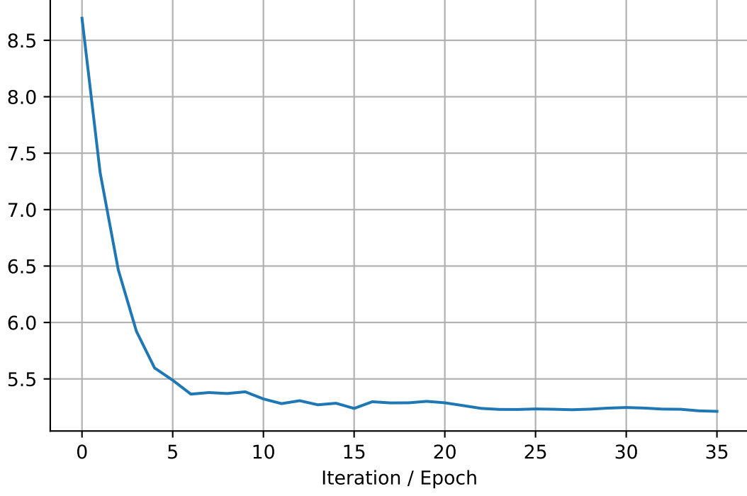
tau2_var
