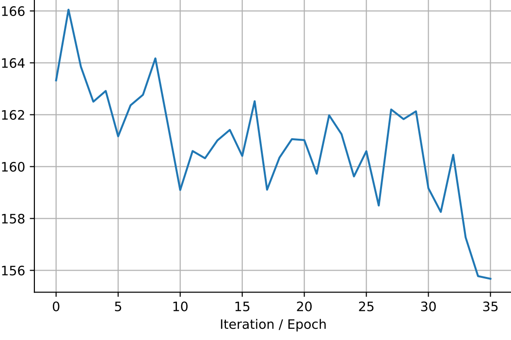
tau2_Eqf2
