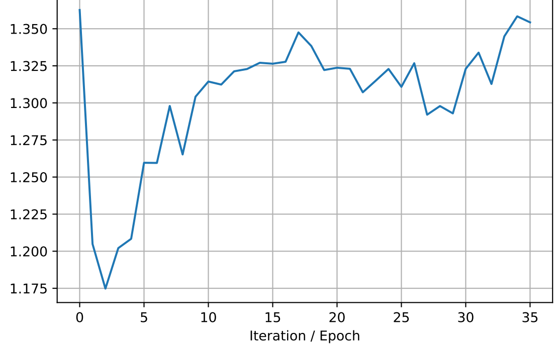
tau1_target_Eqf1
