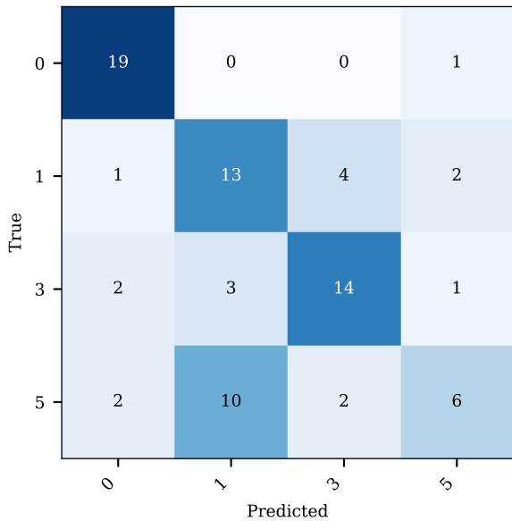
eucl_params (k=10 f1=0.632)
