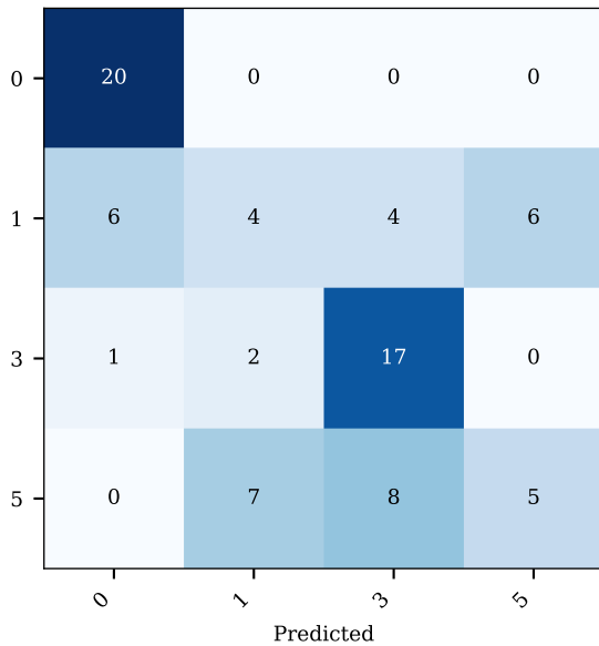
eucl_raw (k=10 f1=0.527)
