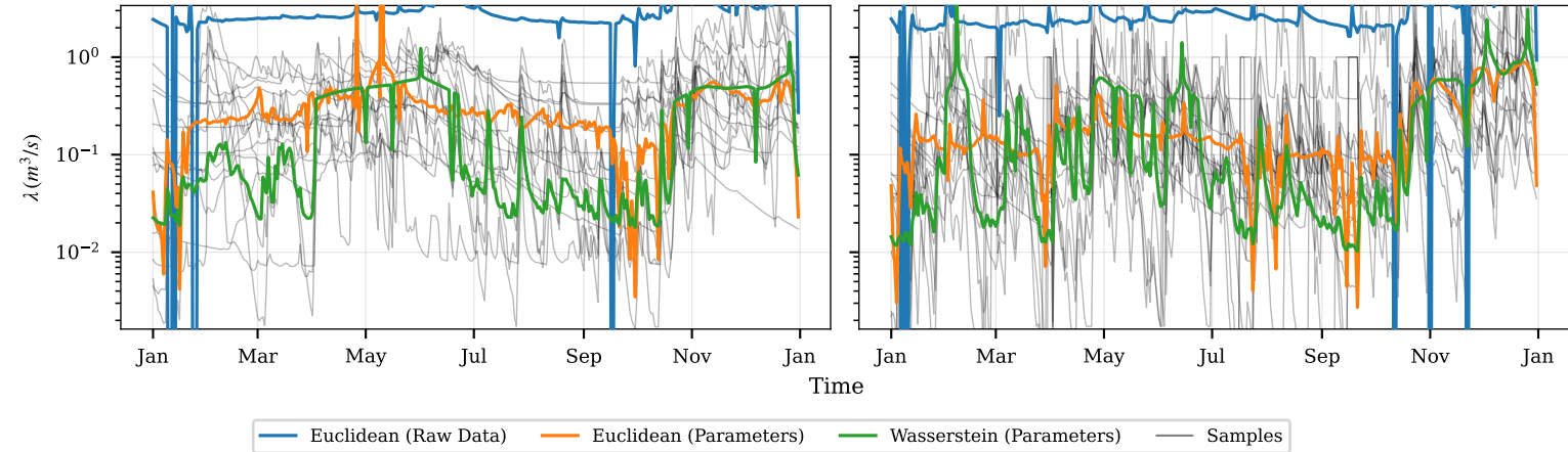
Nivo-pluvial
