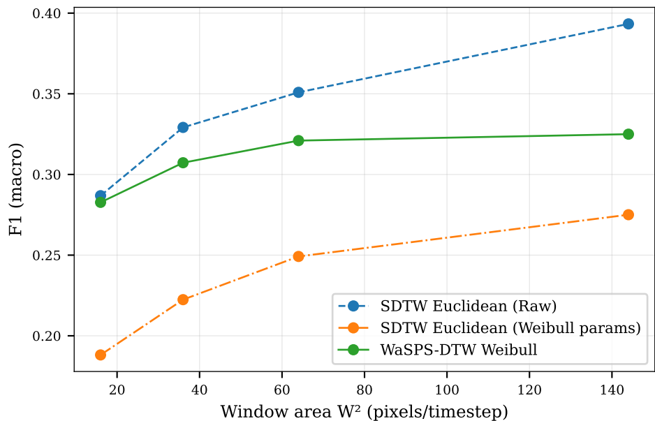
F1 (macro)
