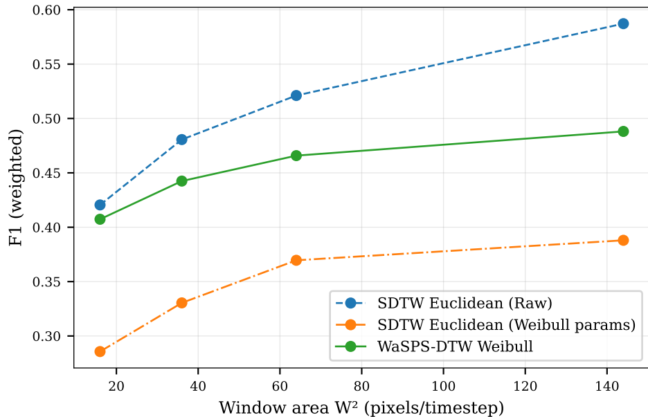
F1 (weighted)
