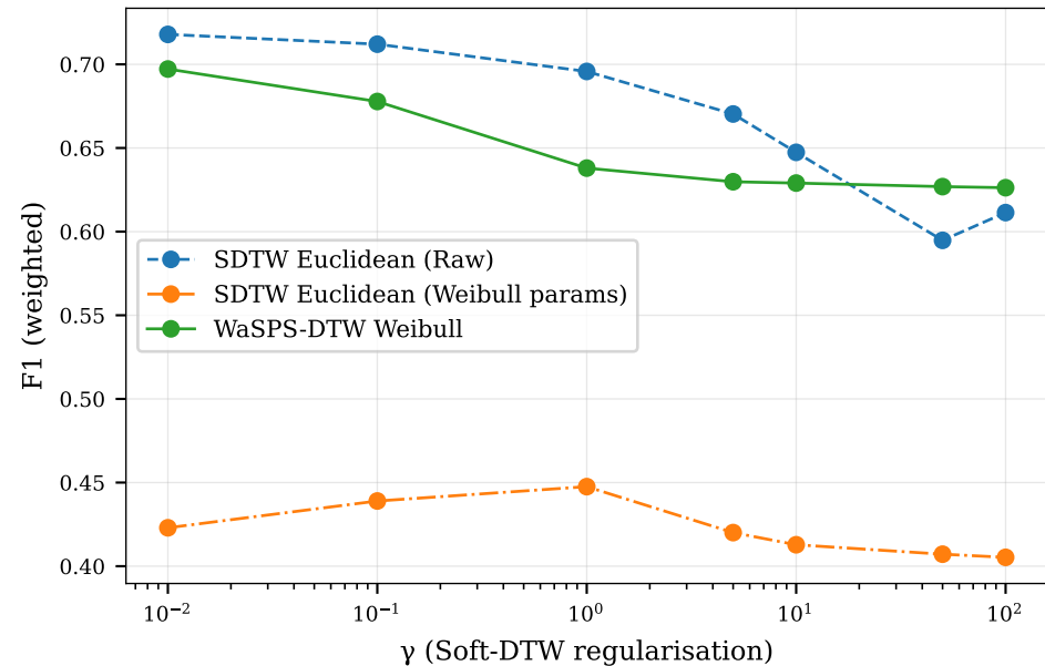
F1 (weighted)
