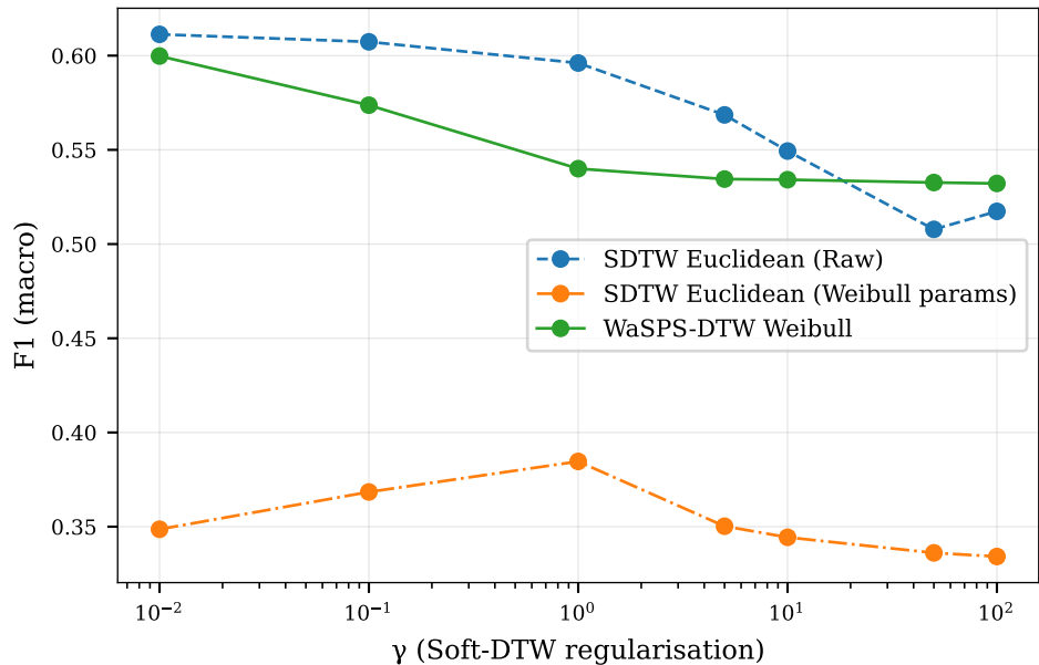
F1 (macro)
