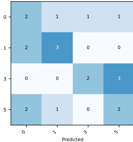
sta f1=0.457
