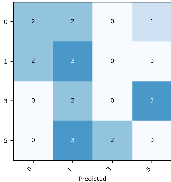
eucl_raw f1=0.211
