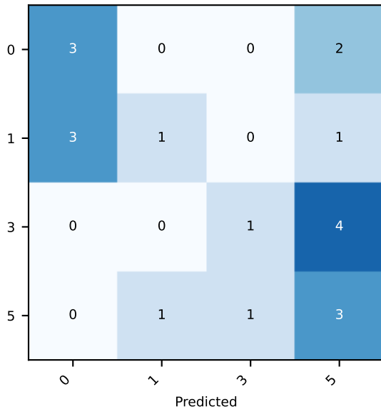
eucl_raw f1=0.379
