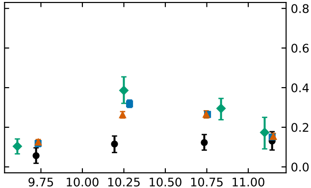
(d) Median \log_{10}(R_{e,r}/\text{kpc})
