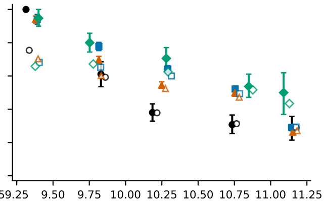
(d) Quenched fraction: BGGs
