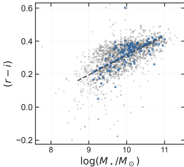
r-i
