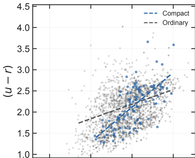
u-r
