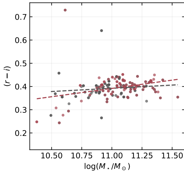
r-i
