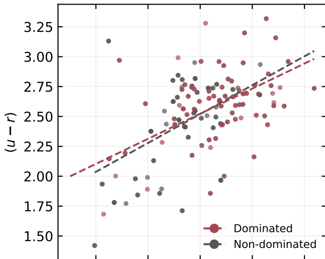
u-r
