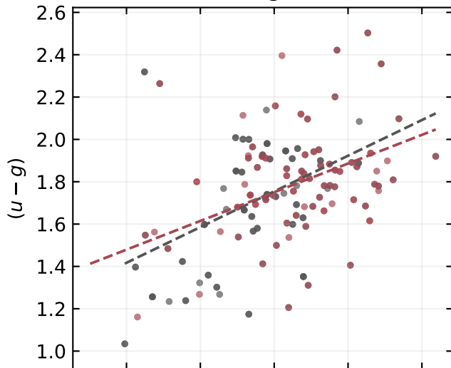
u-g
