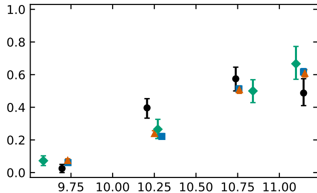
(d) Median \log_{10}(R_e, r/\text{kpc})
