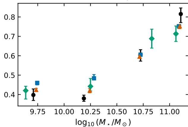
(d) Median \log_{10}(R_e, r/\text{kpc})
