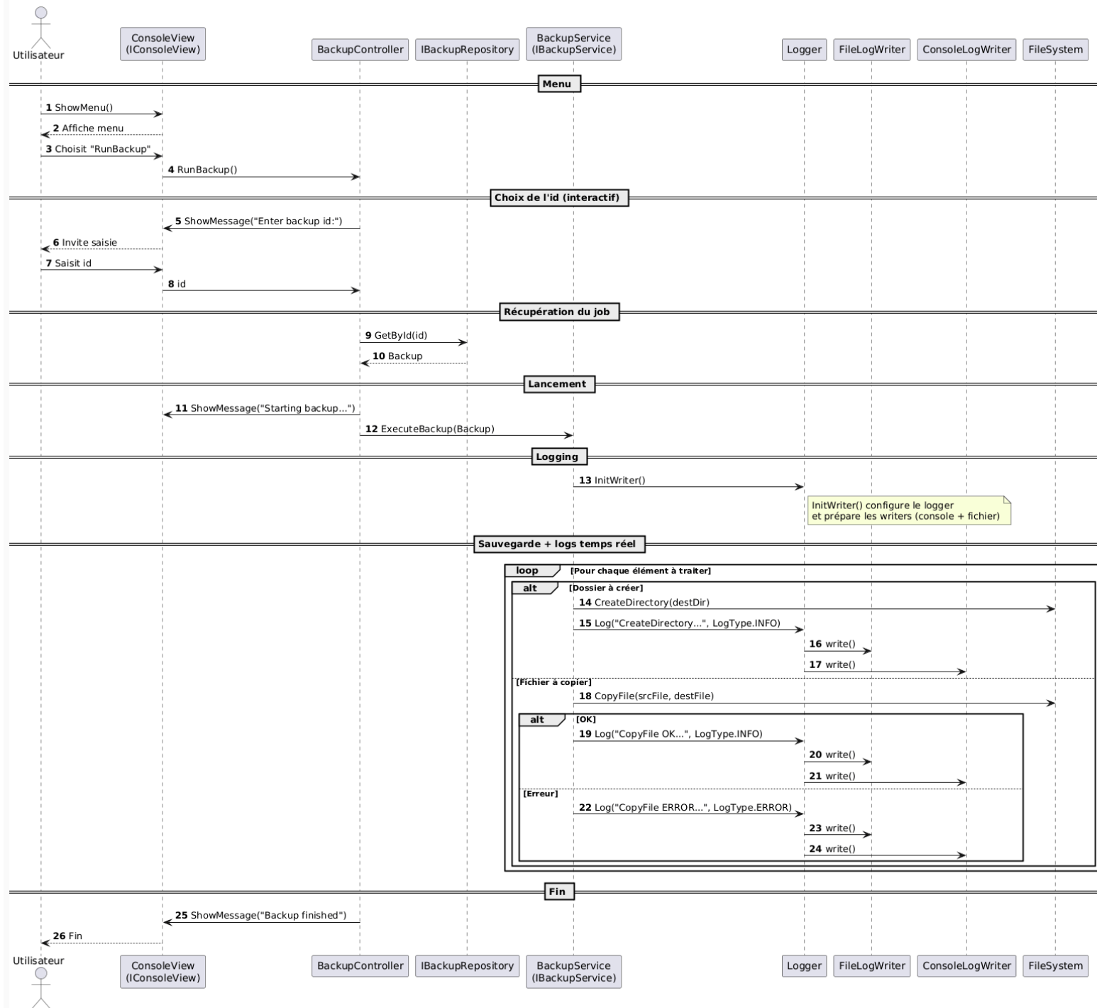
Diagramme de séquence - Execution d'un backup
