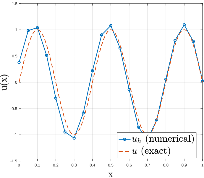
u_h solution for h = 0.05 and nEl = 20
