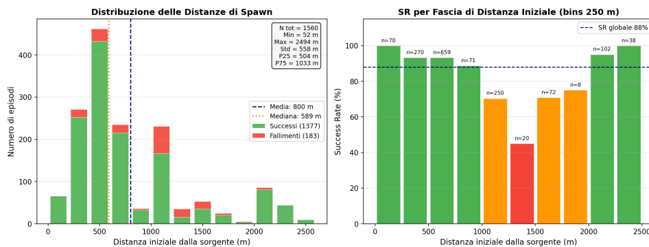
Figura 1: Distribuzione delle distanze iniziali — base .
