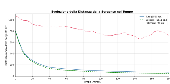
Figura 8: Distanza media dalla sorgente nel tempo — minimal.
