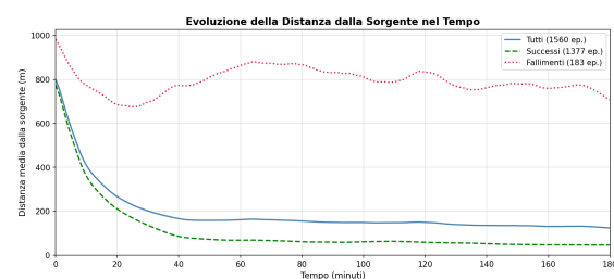
Figura 4: Distanza media dalla sorgente nel tempo — base.
