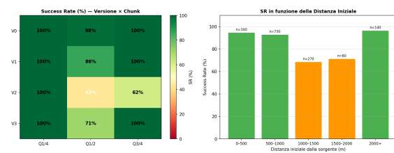
Figura 2: Success rate per scenario — base.
