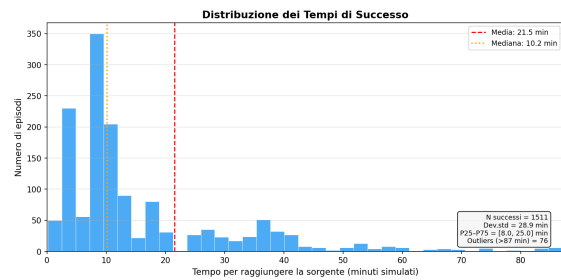
Figura 7: Distribuzione del tempo al successo — minimal.
