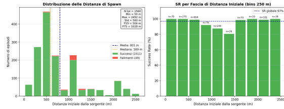
Figura 5: Distribuzione delle distanze iniziali — minimal.
