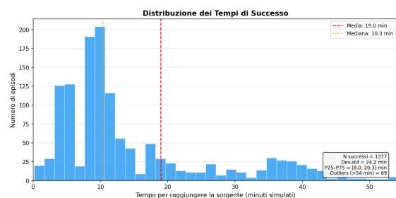
Figura 3: Distribuzione del tempo al successo — base.
