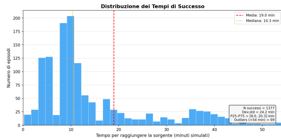
Figura 3: Distribuzione del tempo al successo — base.
