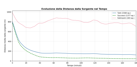
Figura 4: Distanza media dalla sorgente nel tempo — base.
