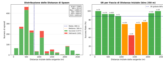
Figura 1: Distribuzione delle distanze iniziali — base.
