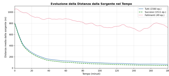
Figura 8: Distanza media dalla sorgente nel tempo — minimal .
