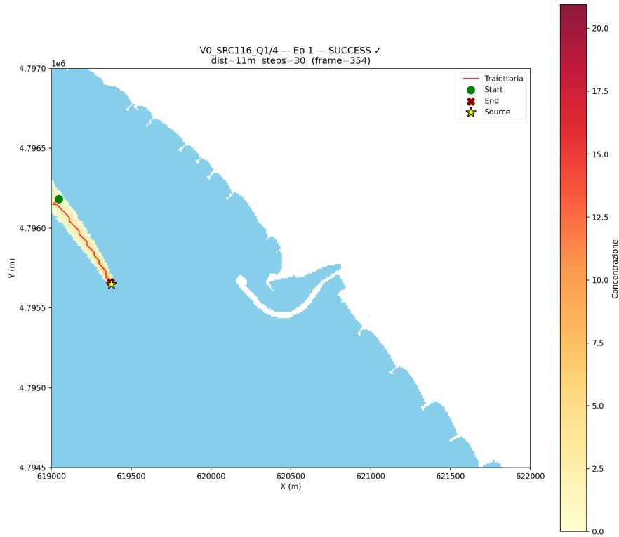
(a) Successo (V0, plume compatto).
