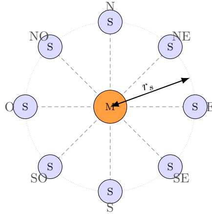
Figura 3.1: Formazione master-slave. L’agente master (M, arancio) occupa il centro; otto agenti slave (S, blu) sono disposti a distanza r_s (il sensor range ) lungo le direzioni cardinali e diagonali. Ogni slave campiona la concentrazione nella propria posizione e la riporta al master; le stesse otto direzioni sono anche le azioni di movimento disponibili.
