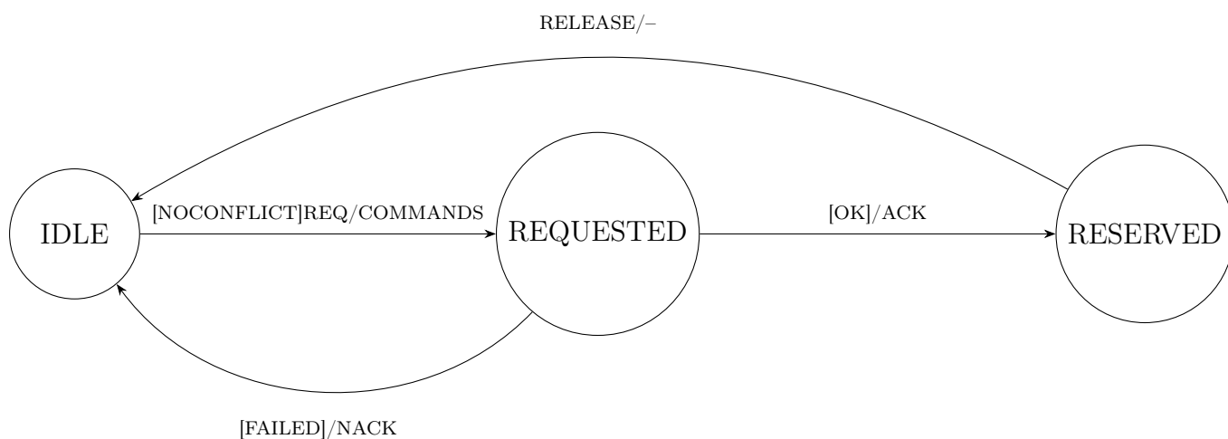
Figura 3: Macchina a stati ITINERARIO
