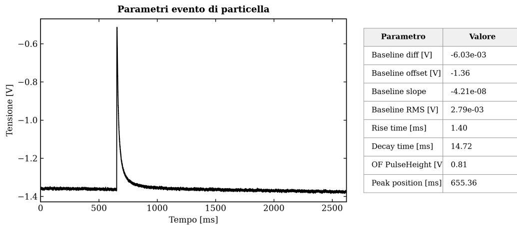
Figura 3.2: Esempio di traccia di particella registrata nel cristallo (a sinistra) e relativa tabella dei parametri di forma calcolati (a destra). (Sistemare unità di misura!!!!)
