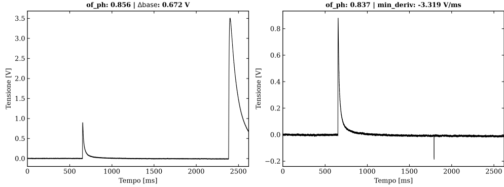
Figura 3.5: Esempi di eventi fisici scartati dai tagli preliminari a causa di anomalie di baseline e problemi alla linearità del rivelatore: in particolare si nota il primo evento soggetto ad una elevata baseline difference dovuta ad un secondo evento verificatosi nella stessa finestra, mentre nel secondo caso una spike negativa dovuta probabilmente ad un'anomalia dell'elettronica.
