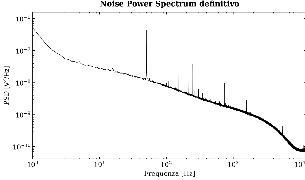
Figura 3.4: Noise Power Spectrum ottenuto dalla media e normalizzazione di circa 1000 eventi di rumore depurati con fit di terzo grado.
