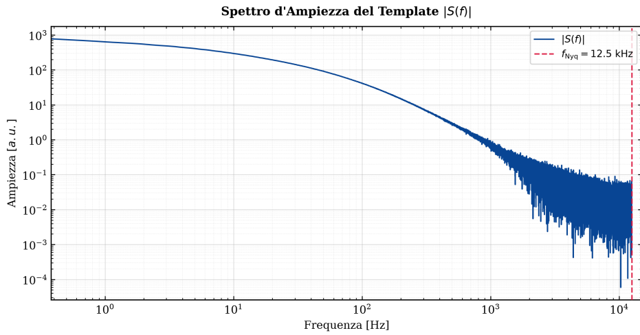
Figura 3.7: Spettro di Fourier S(f) del template fononico.
