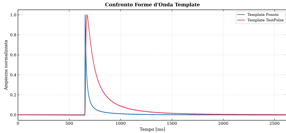
Figura 3.8: Confronto normalizzato tra il template di particella ( ^{55}\text{Fe} ) e il template ricavato dai TestPulses: l'impulso da particella presenta un tempo di salita più rapido.
