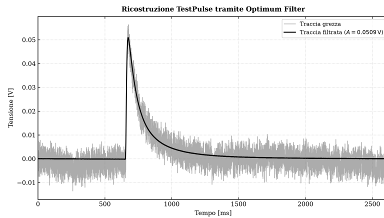
Figura 3.10: Applicazione dell'Optimum Filter a un TestPulse a bassa energia: confronto tra traccia grezza (grigio) e ricostruzione ottenuta scalando il template sull'ampiezza stimata (nero).
