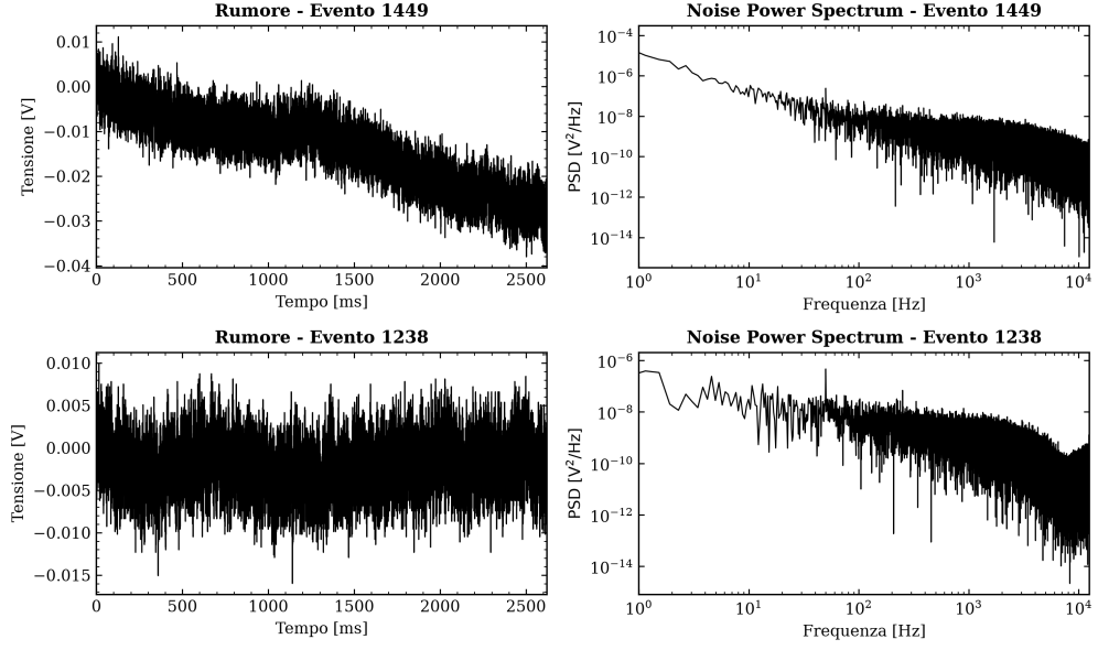
Figura 3.3: Confronto tra due tracce di rumore: l'evento superiore risente di una deriva di baseline che produce un gradino tra i margini, generando nello spettro un'iniezione fittizia di potenza a bassa frequenza; l'evento inferiore, piatto e stazionario, restituisce il profilo indisturbato del rumore.
