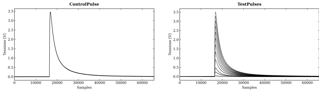
(a) Impulso a 20 V (ControlPulse).
