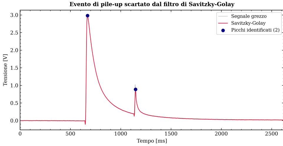
Figura 3.6: Identificazione del pile-up tramite Savitzky-Golay: la curva smussata (in rosso) permette all'algoritmo di intercettare il secondo massimo locale ed escludere la traccia dal calcolo del template.
