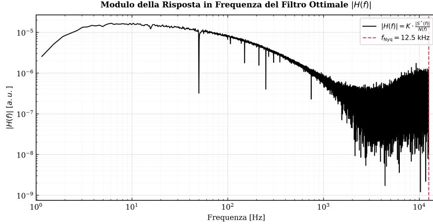
Figura 3.9: Modulo della funzione di trasferimento H(f) dell'Optimum Filter per un evento di particella: si nota l'accentuata soppressione in corrispondenza del rumore di rete (50 Hz) e alle alte frequenze.
