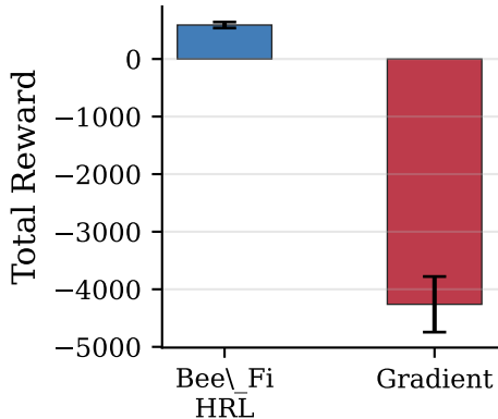
Episodic Reward
