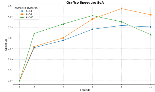
Figure 5. Speedup della versione SoA all'aumentare del numero di cluster.
