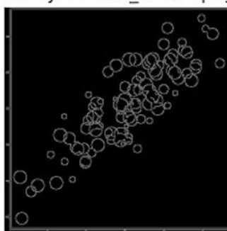
Canny: bubble_00004.png
