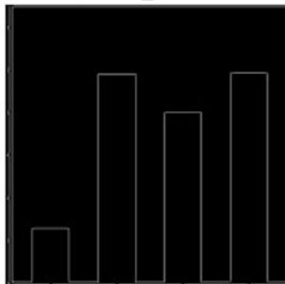
Canny: bubble_00004.png
