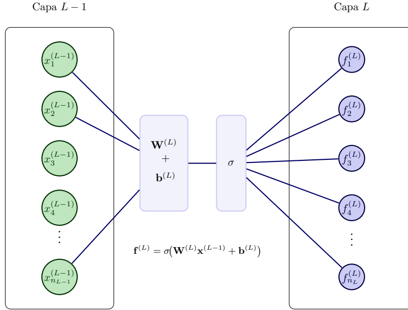
Figura 3.3: Capa de una red neuronal con múltiples neuronas en la capa L .
