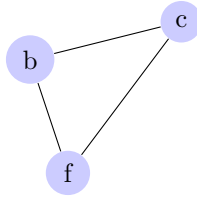
Figura 7: Ejemplo de una gráfica inducida
