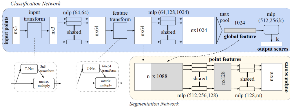
Figura 9: Arquitectura PointNet [?]
