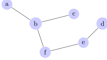
Figura 6: Ejemplo de una gráfica H que abarca G
