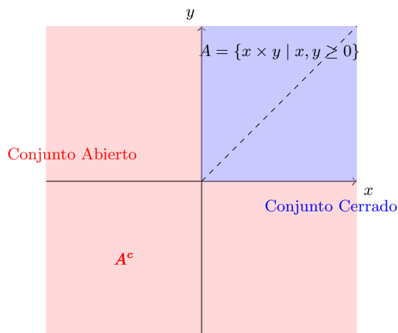
Figura 1: Ilustración del subconjunto A
