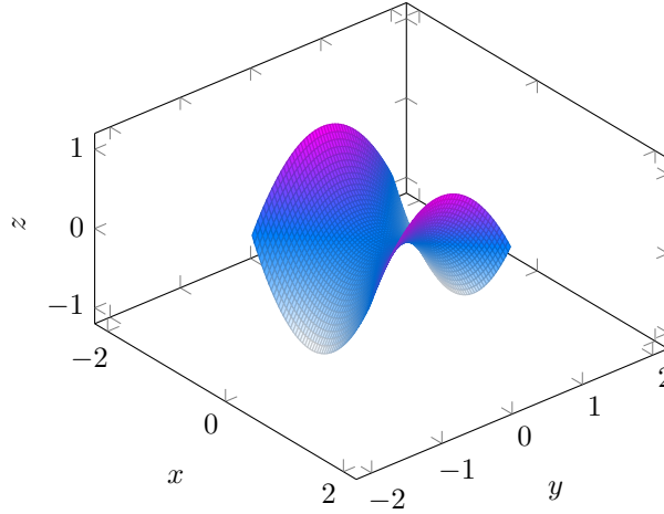
Figura 3: Ejemplo de superficie en \mathbb{R}^3 comúnmente conocida como "Silla de Montar"
