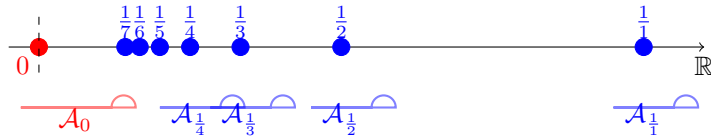
Figura 2: Ilustración de la compactidad del espacio X
