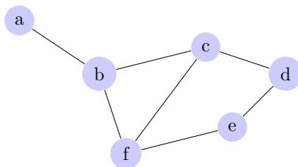
Figura 4: Ejemplo de gráfica simple G
