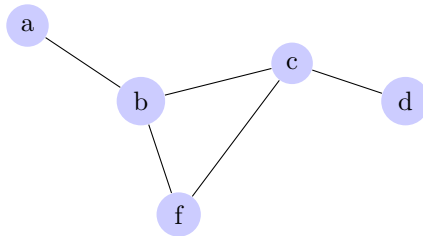
Figura 5: Ejemplo de subgráfica de G
