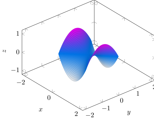
Figura 1: Ejemplo de superficie en \mathbb{R}^3 comúnmente conocida como "Silla de Montar"
