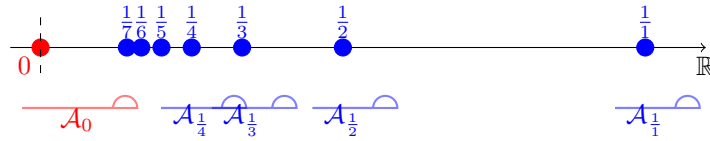
Figura 2.2: Ilustración de la compacidad del espacio X
