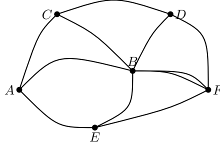
Figura 2.5: Ejemplo de triangulación en una superficie
