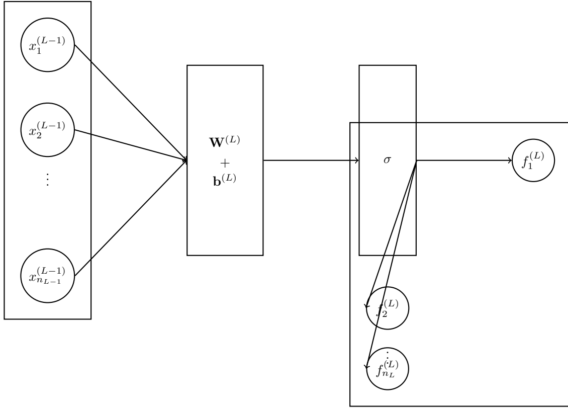
Figura 3.2: Capa de una red neuronal
