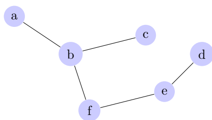
Figura 2.8: Ejemplo de una gráfica H que abarca G
