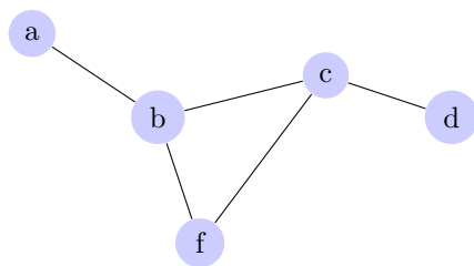
Figura 2.7: Ejemplo de subgráfica de G
