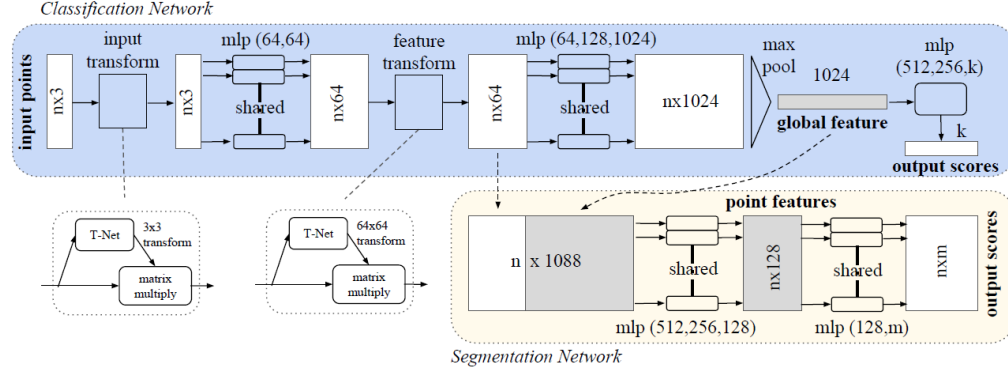
Figura 5.1: Arquitectura PointNet [8]
