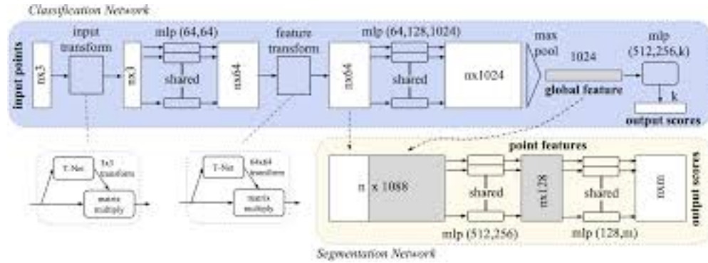
Figura 7: Arquitectura PointNet [?]
