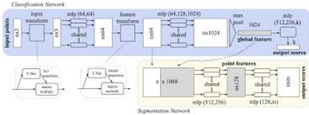
Figura 7: Arquitectura PointNet [7]
