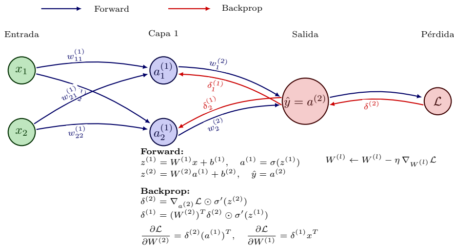
Figura 3.6: Backpropagation: forward (azul) y backward (rojo) con trayectorias separadas mediante desplazamiento de anclajes.
