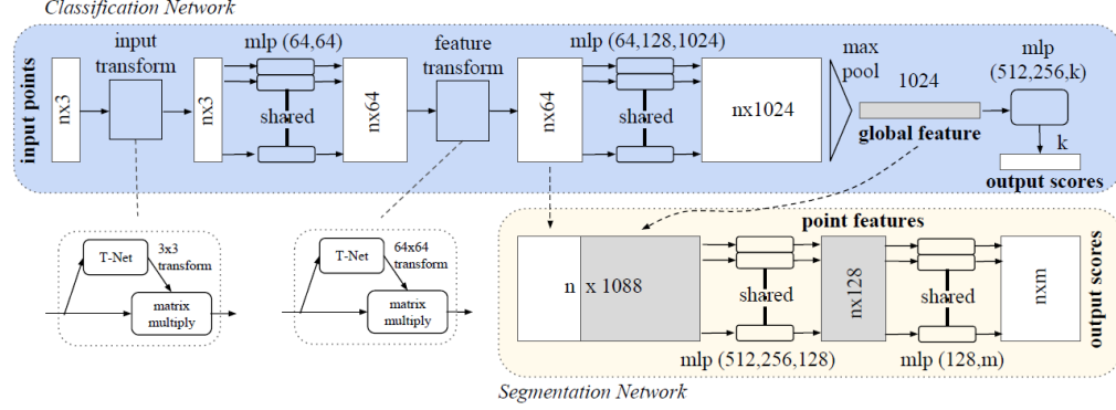
Figura 5.1: Arquitectura PointNet [?]
