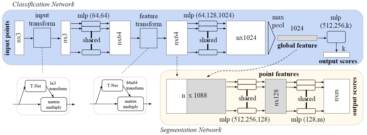
Figura 7: Arquitectura PointNet [?]
