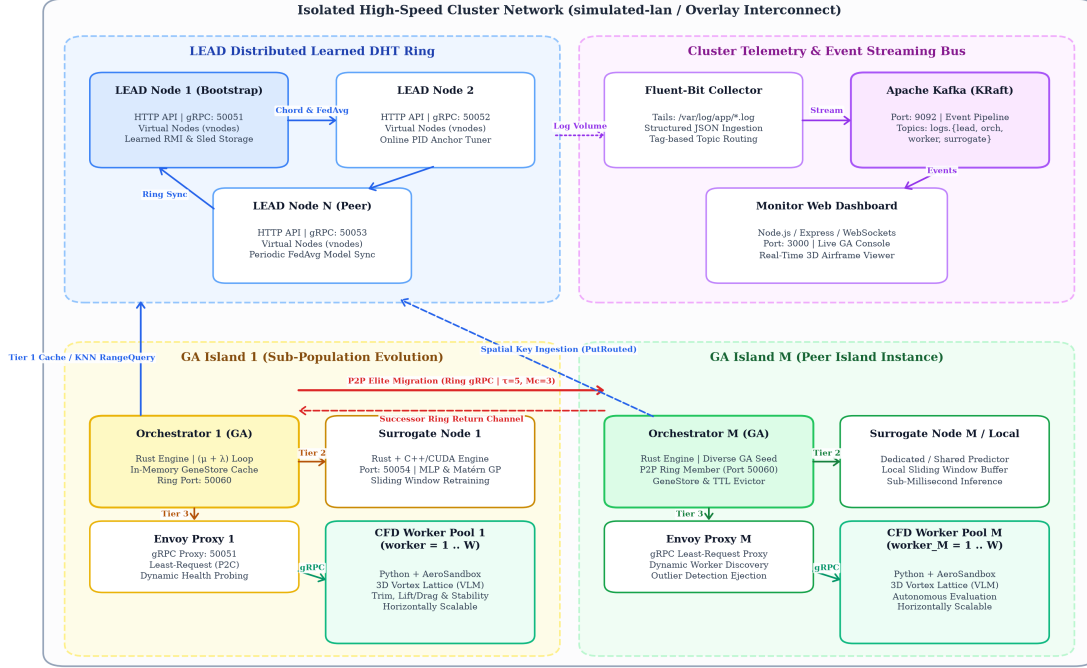
Σχήμα 3.1: Συνολική αρχιτεκτονική τοπολογία του κατανεμημένου συστήματος: Δακτύλιος νήσων Orchestrator (Chord Ring), δακτύλιος LEAD DHT με χωρική ευρετηρίαση Hilbert, επιταχυντής υποκατάστασης Surrogate Node, ισοσταθμιστής φορτίου Envoy και συστοιχία υπολογιστικών εργατών AeroSandbox CFD.
