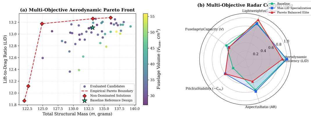
Σχήμα 5.22: Πολυ-αντικειμενική αεροδυναμική ανάλυση Pareto: (α) Μέτωπο Pareto μεταξύ αεροδυναμικής απόδοσης ( L/D ) και δομικής μάζας, και (β) 5-αξονικό διάγραμμα ραντάρ συγκρίνοντας τη βασική διαμόρφωση, την εξειδίκευση μέγιστου L/D και την ισορροπημένη ελίτ λύση.
