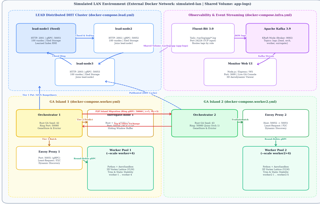
Σχήμα 3.1: Συνολική αρχιτεκτονική τοπολογία του κατανεμημένου συστήματος: Δακτύλιος νήσων Orchestrator (Chord Ring), δακτύλιος LEAD DHT με χωρική ευρετηρίαση Hilbert, επιταχυντής υποκατάστασης Surrogate Node, ισοσταθμιστής φορτίου Envoy και συστοιχία υπολογιστικών εργατών AeroSandbox CFD.
