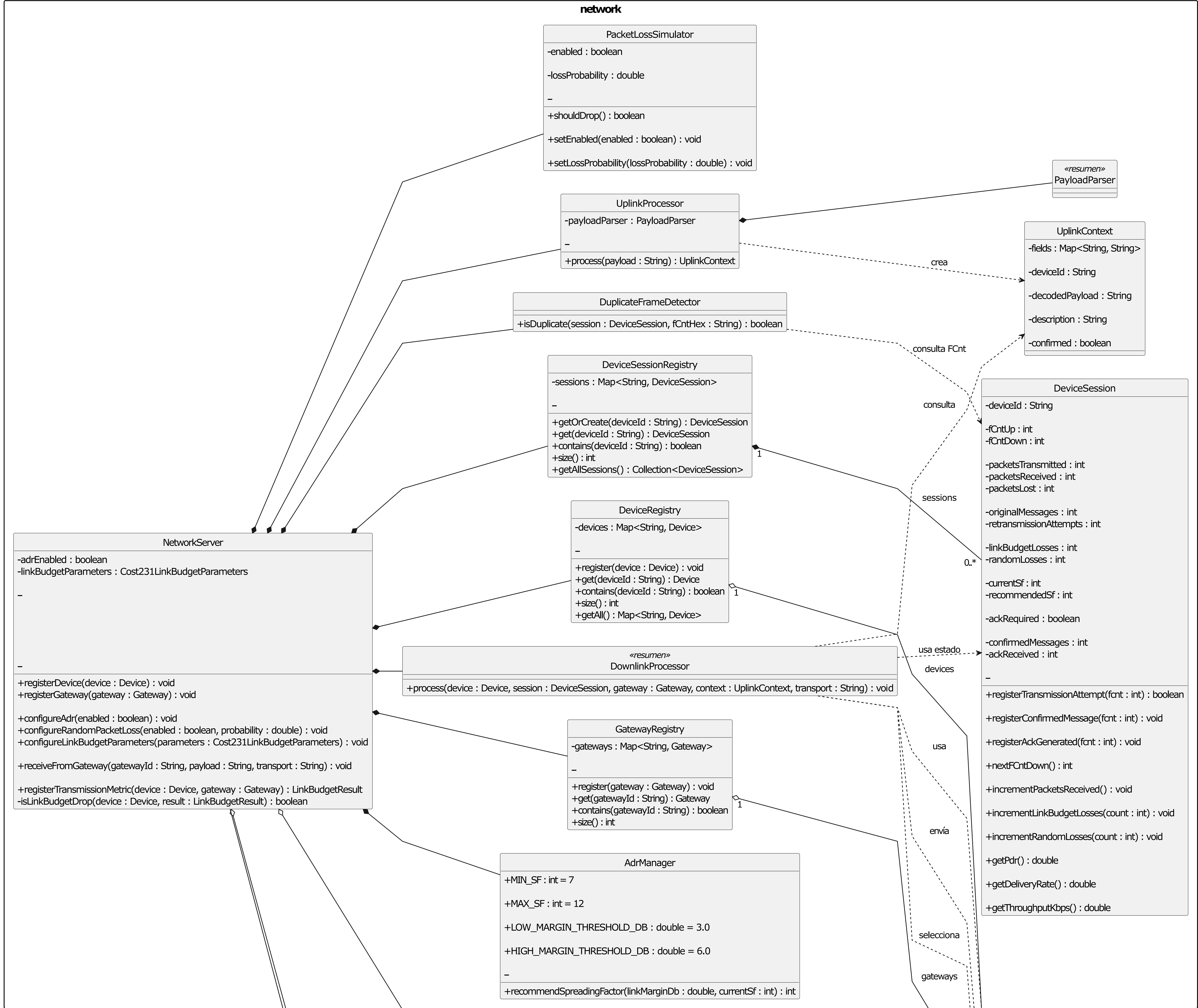
Diagrama de clases — Procesamiento del Network Server
