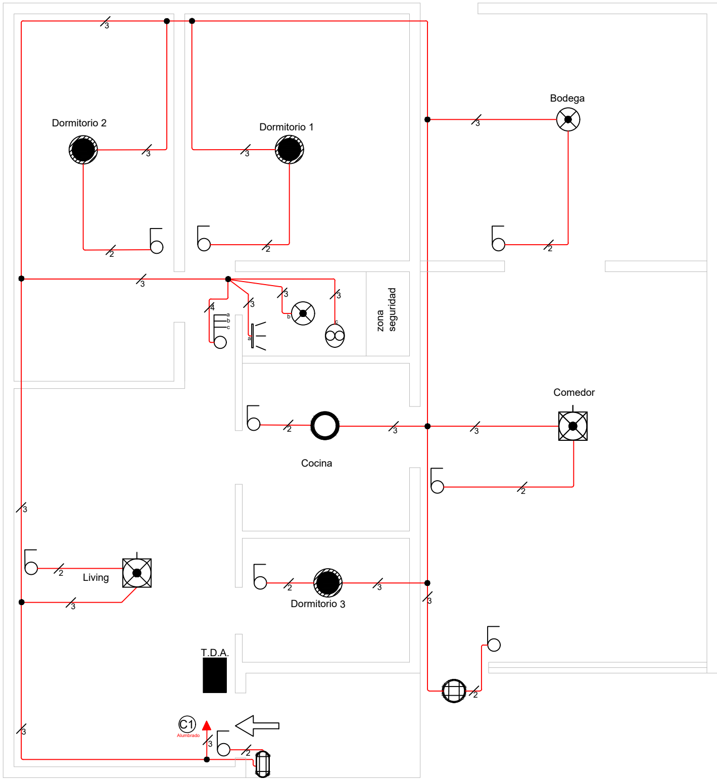
PLANTA DE ALUMBRADO — C1 — E: 1/50
