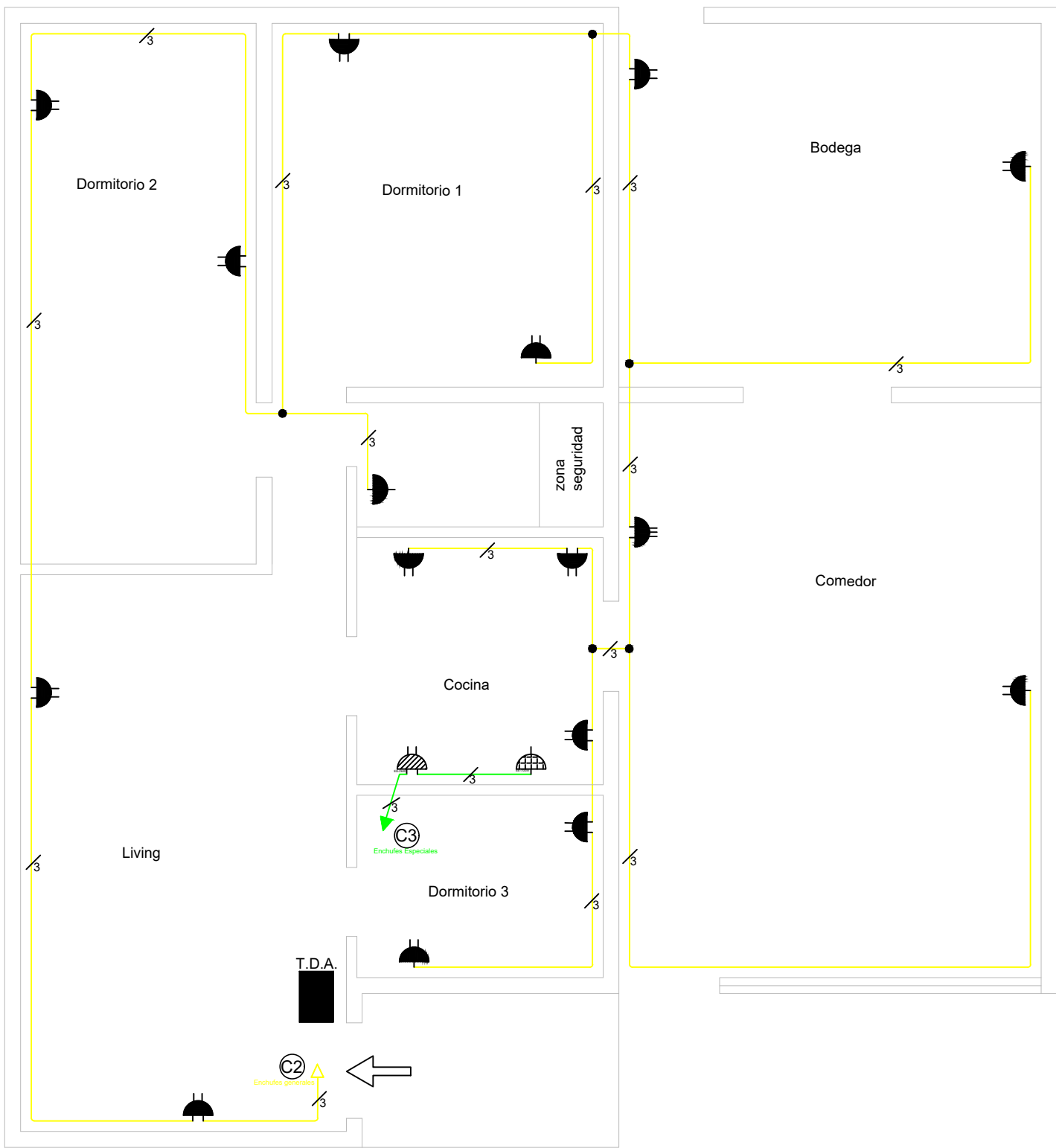
PLANTA DE ENCHUFES — C2 y C3 — E: 1/50
