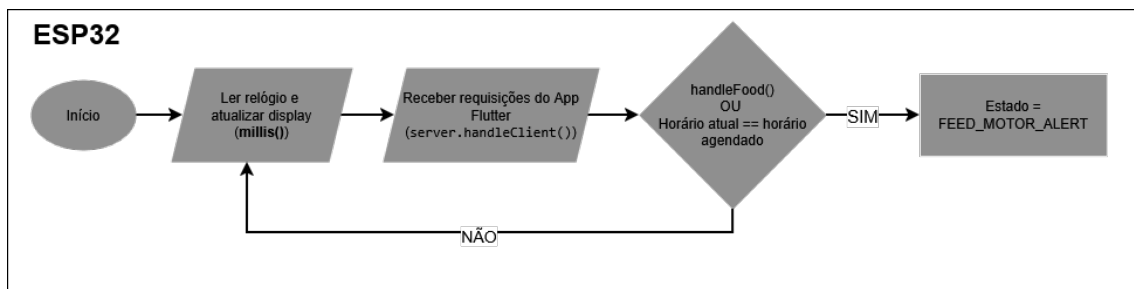
Figura 3. Fluxograma Dispositivo - Cadeia de Alimentação
