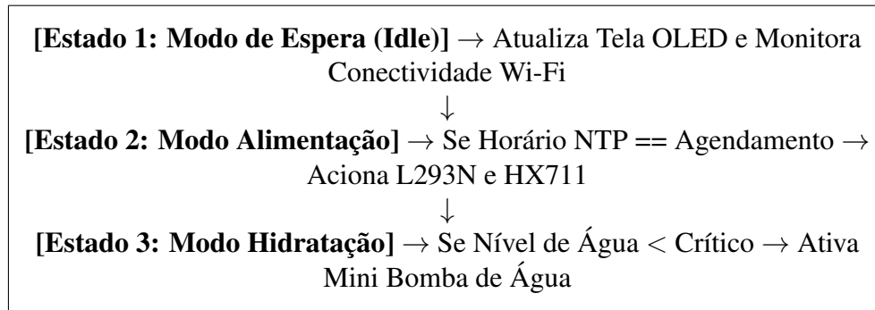
Figura 1. Representação estrutural do fluxograma de estados do firmware.
