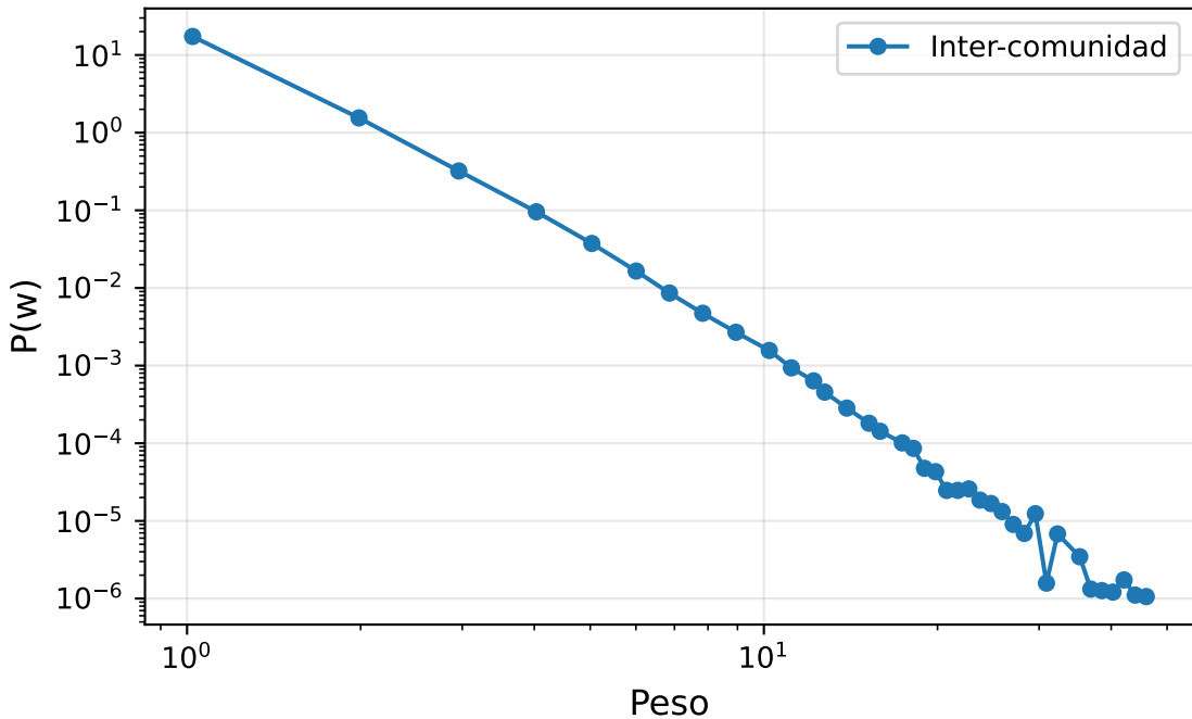
Distribución de pesos inter-comunidad (926501 aristas)
